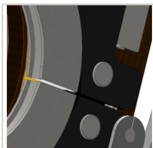
Montaggio delle morse senza utensili
