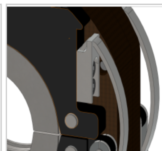
Sistema ad effetto molla regolabile: tiene conto dell'ovalizzazione dei tubi
